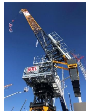
Wippkran SLH 70.4. Mit nur 4 m Radius der Verstellausleger mit dem wohl geringsten Platzbedarf.
