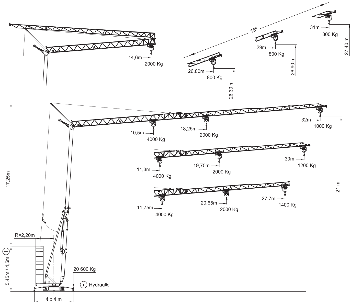
Weight ballast / Gewicht Ballast
